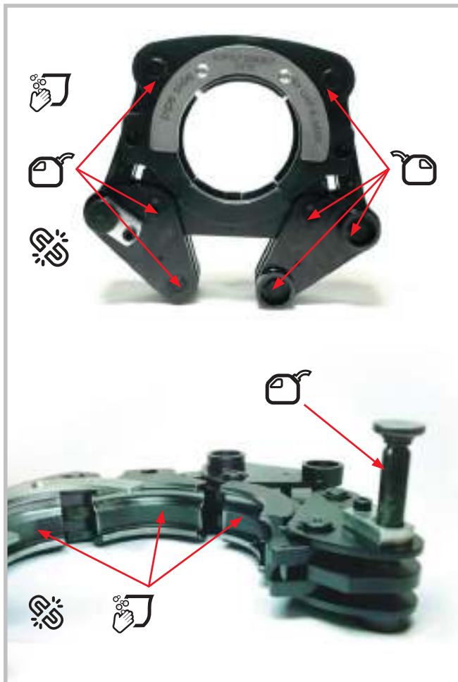
Рис.18. Инструмент Klauke.
